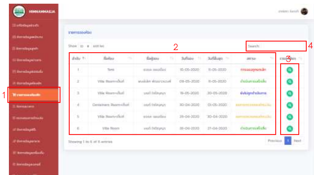
ภาพที่ ก.16 แสดงหน้าจอรายการจองห้องพัก
